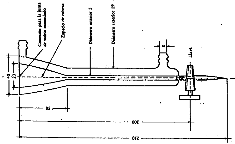
Figura 3 Microcolumna tipo (dimensiones en milímetros)
