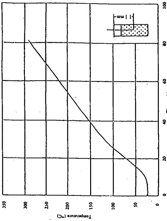
Figura 3 Calibración de la velocidad de calentamiento en el ensayo de sensibilidad térmica
