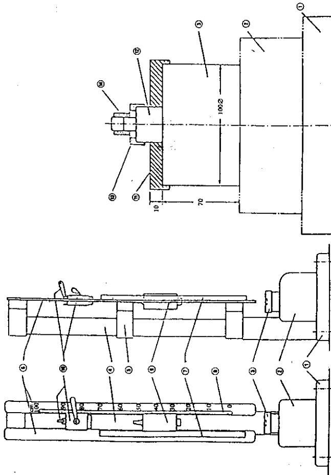
Fig. 4a Martinete, vista general frontal y lateral
