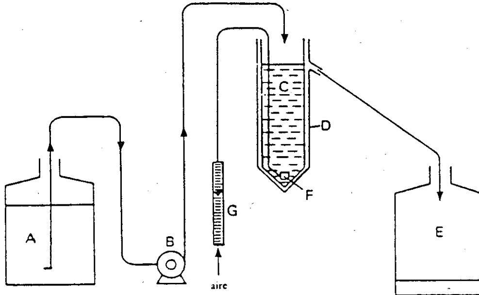
Equipo utilizado para valorar la biodegradabilidad
