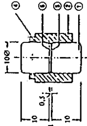
Fig. 4d Dispositivo de choque para sustancias líquidas
