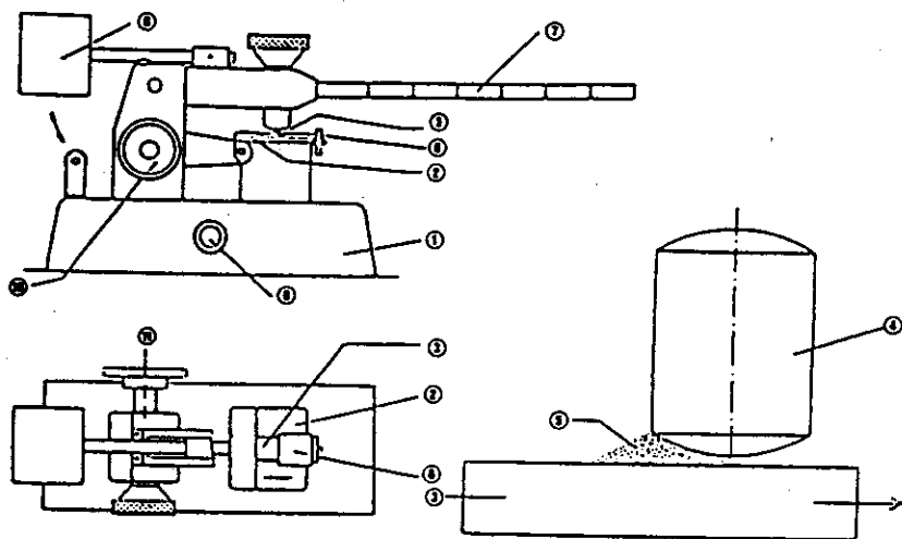
Fig. 5a Equipo de fricción: vista de frente y planta
